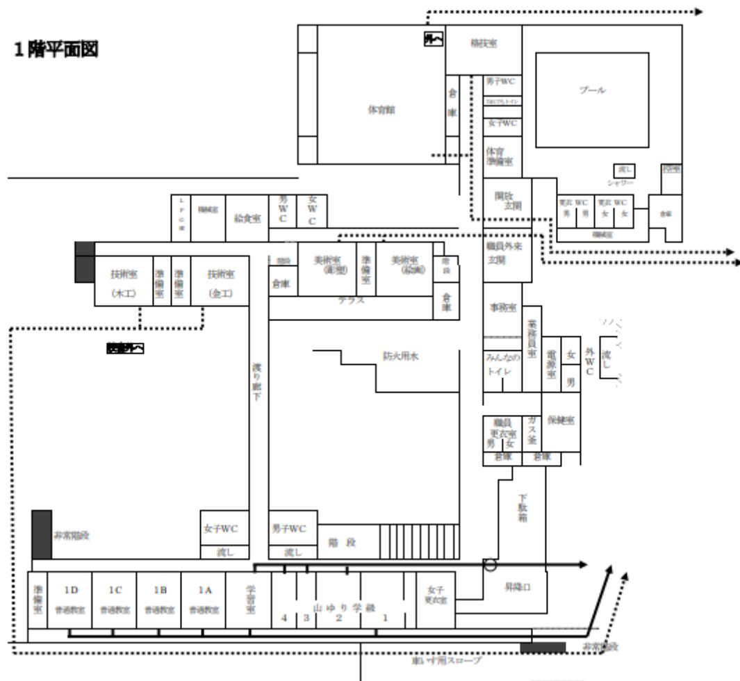
避難経路図
