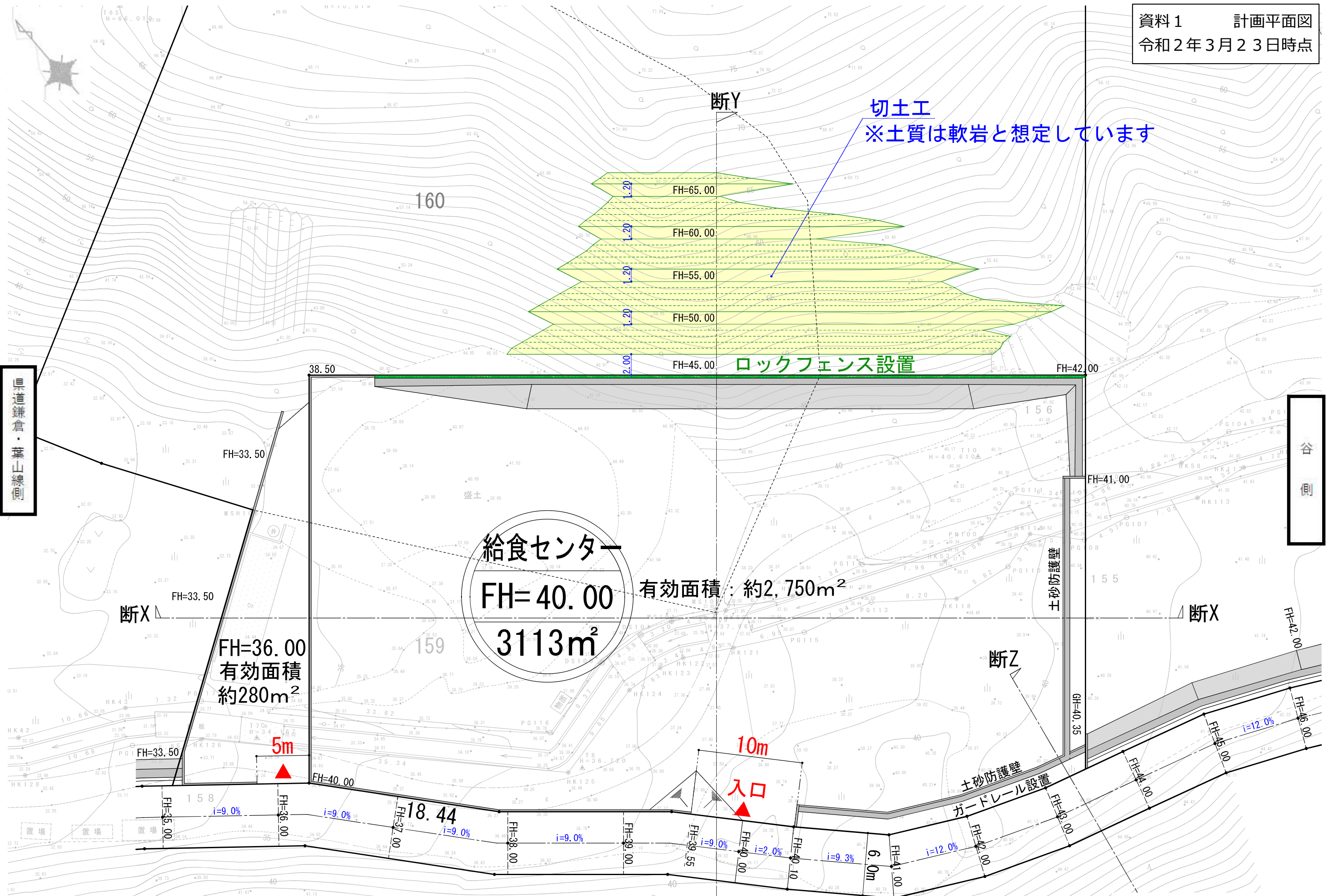
平面図(給食センター) S=1/300
