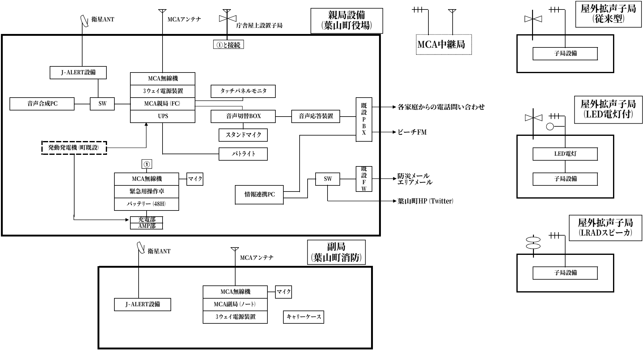
防災行政無線システム構成図
