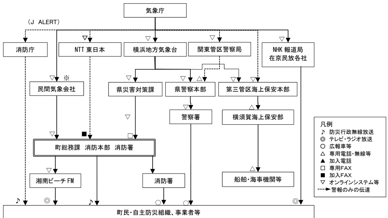
〈伝達系統図〉
