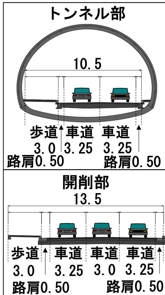
標準横断図
