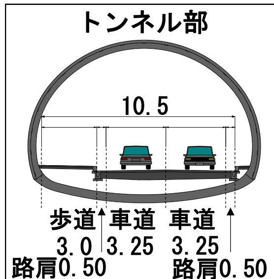
標準横断図
