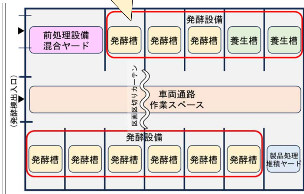
発酵棟内概略配置図
